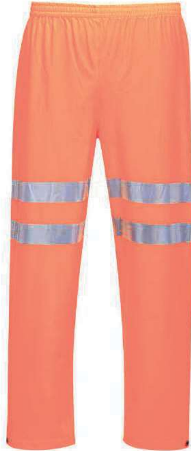
RT51 ΑΝΑΚΛΑΣΤΙΚΟ ΑΔΙΑΒΡΟΧΟ ΠΑΝΤΕΛΟΝΙ SEALTEX ULTRA EN ISO 20471 ΚΛΑΣΗ 2 EN 343 ΚΛΑΣΗ 3:2 X WP 5,000MM, MVP 3,000G/M 2 /24HRS
